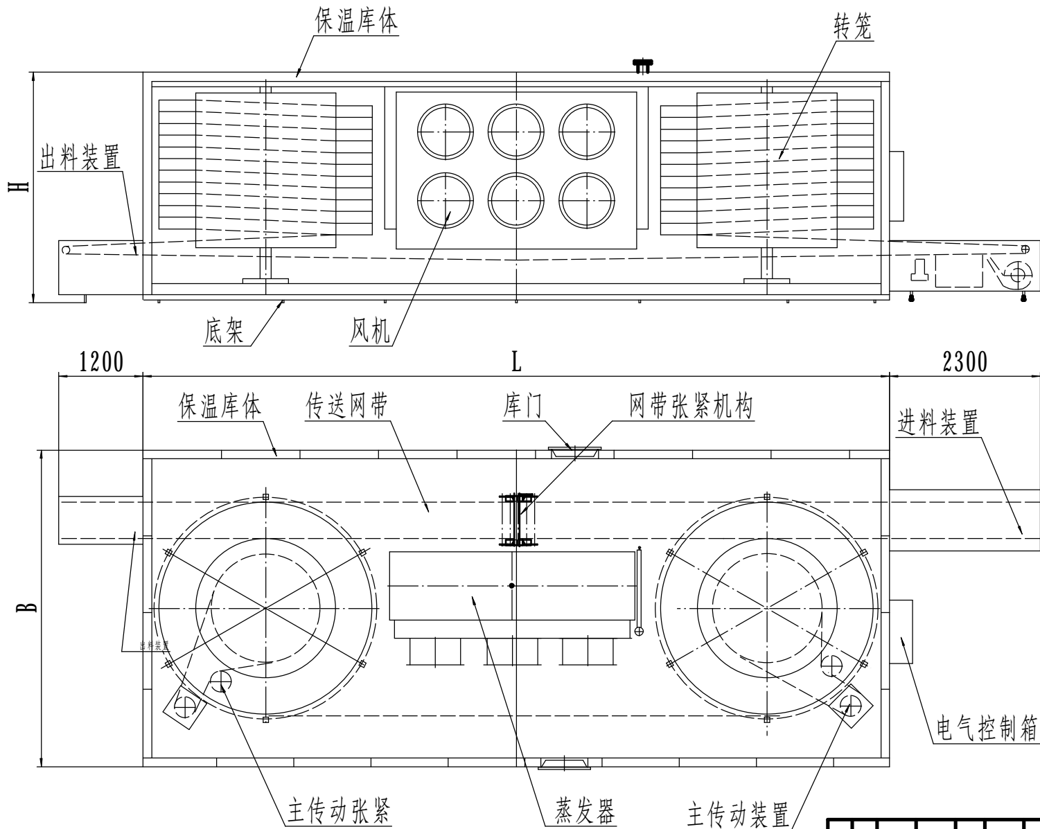
SD-双螺旋速冻装置示意图
