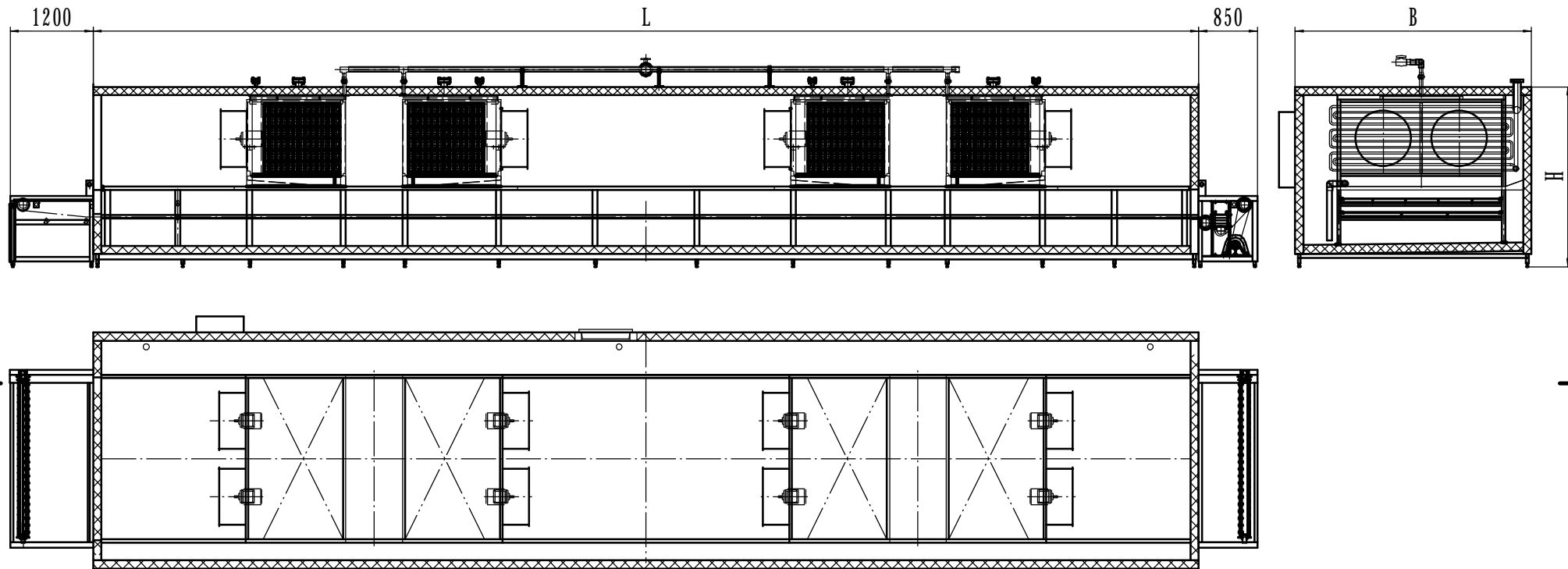
TWS网带速冻机示意图
